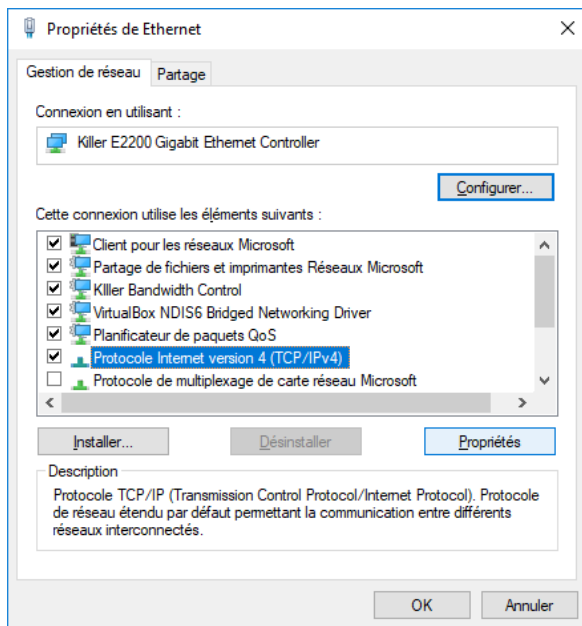
Illustration 26: sélectionner IPv4
